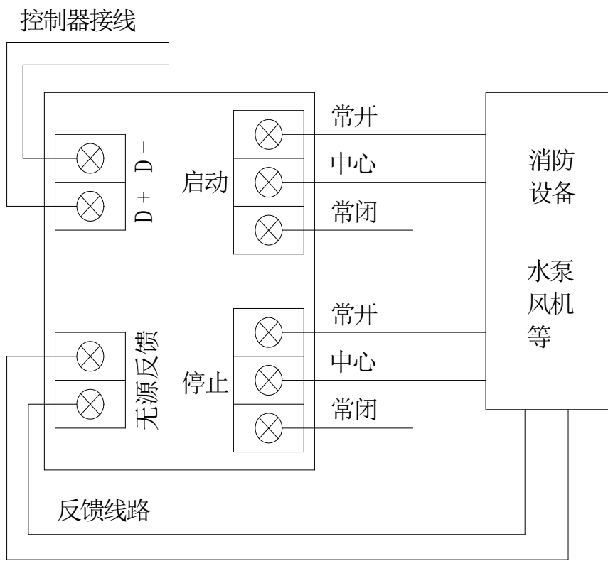
直接启动装置示意图
